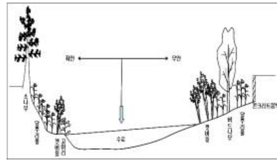
실내작업을 거쳐 완성된 식생단면도
